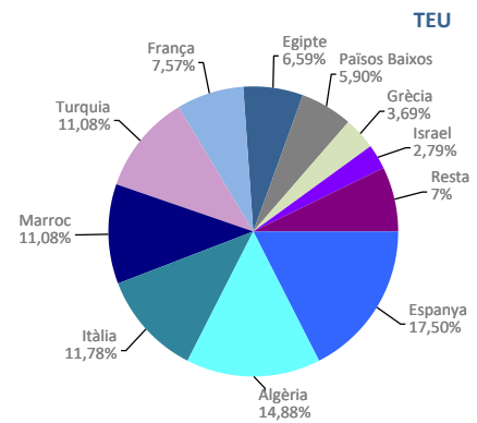
Principals països
